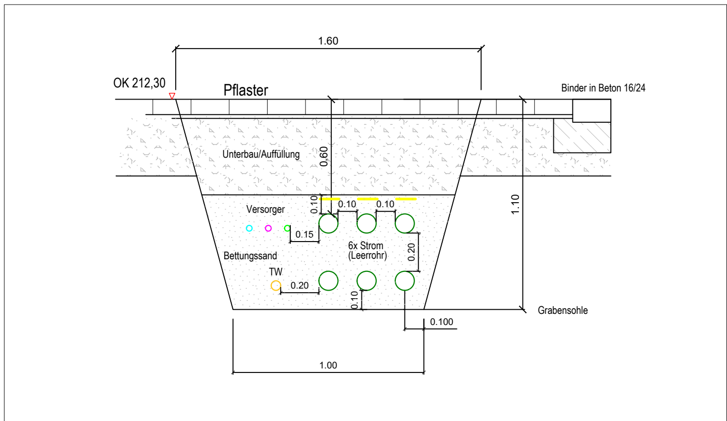
Schnitt 1 / Grabenprofil A Entlang des Gebäudes
