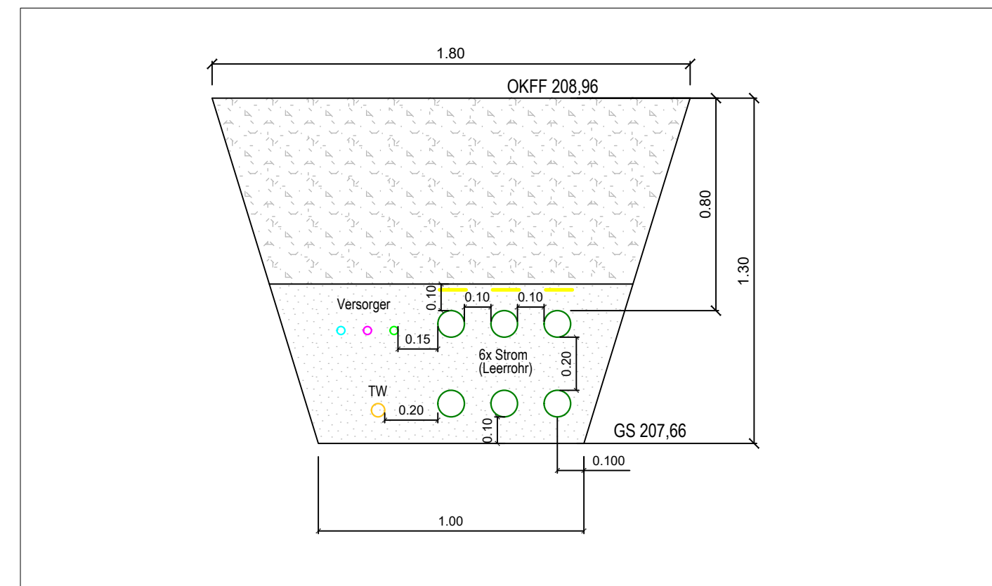
Schnitt 3 / Grabenprofil B Anschluss Gebäude
