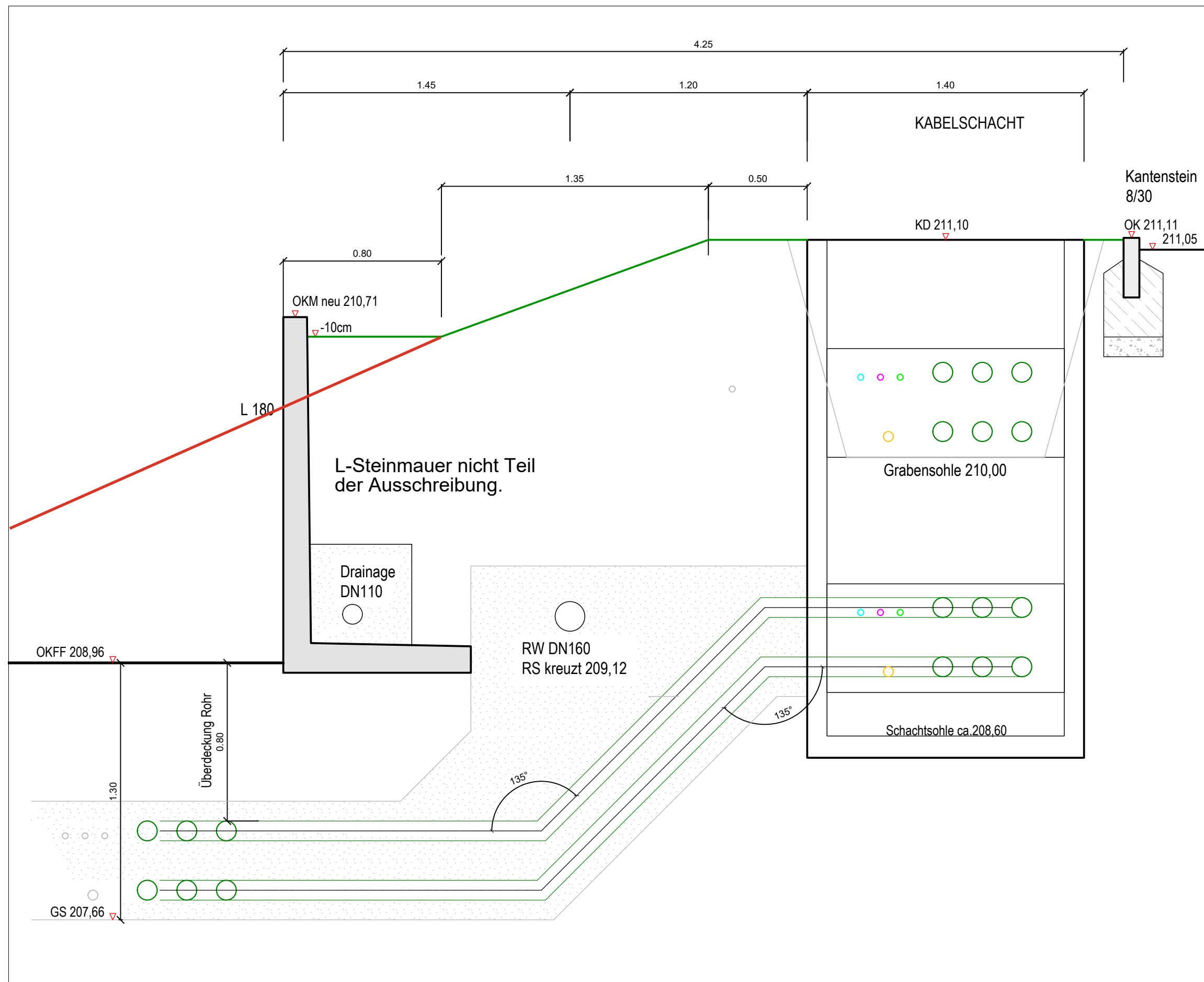
Schnitt 2: Kabelschacht / Anschluss Gebäude
